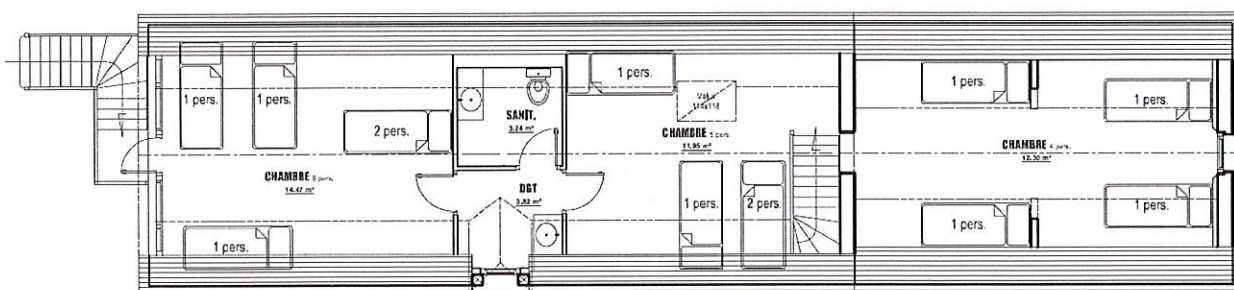
PLAN - ETAGE
