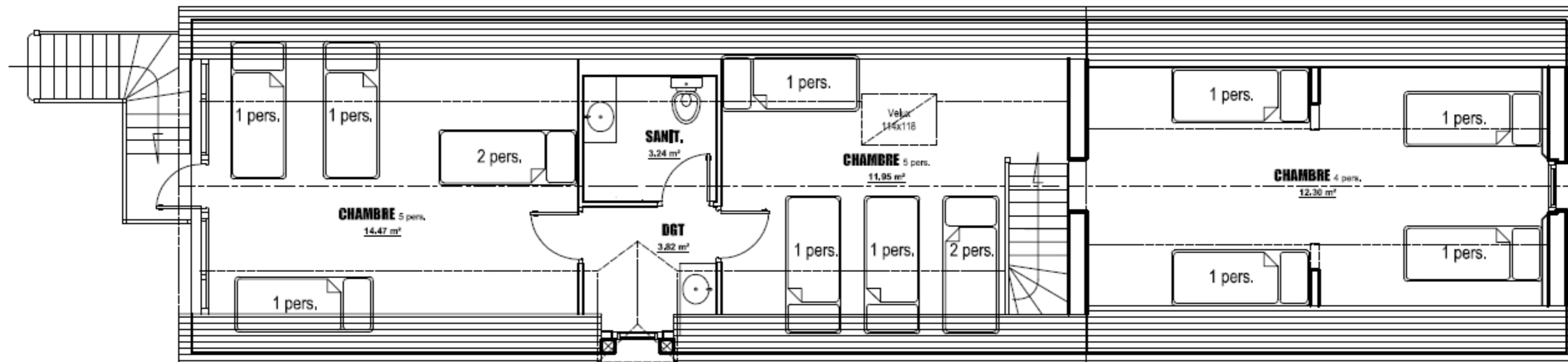
PLAN - ETAGE
