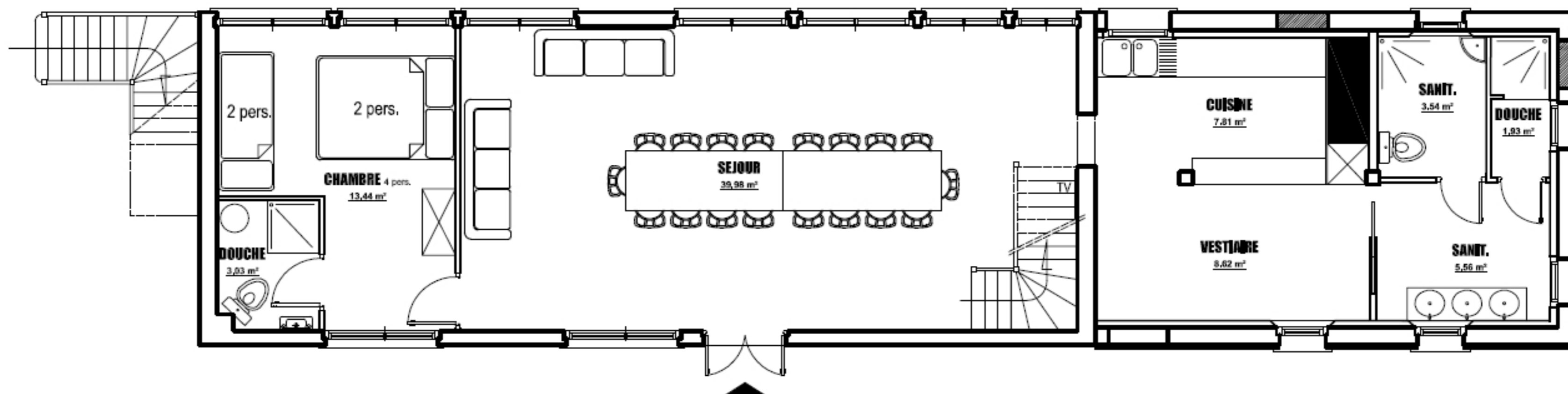
PLAN - REZ de CHAUSSEE
